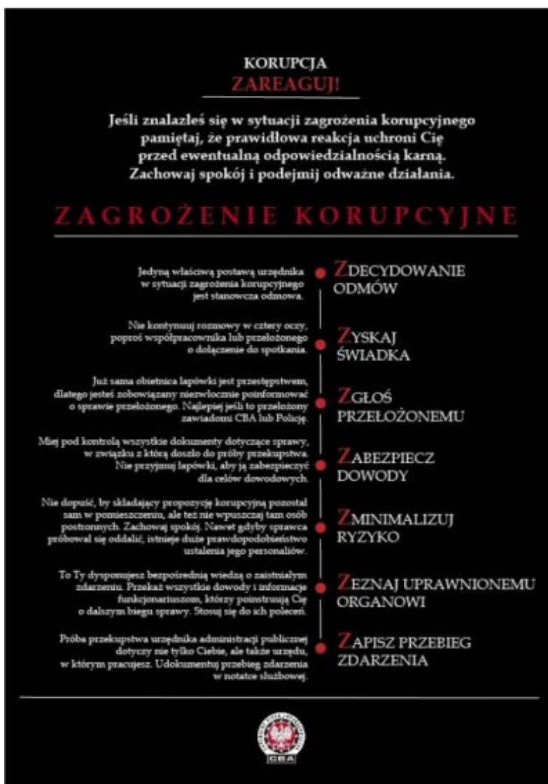
Algorytm
